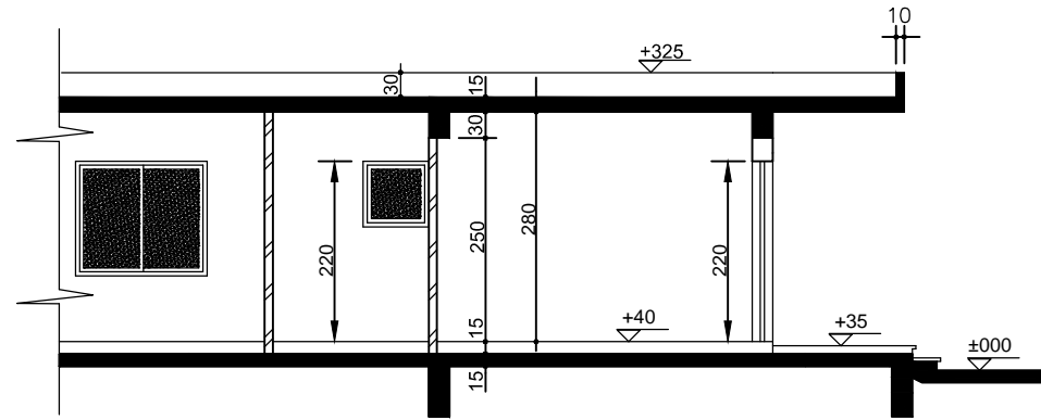
ΤΥΠΙΚΗ ΤΟΜΗ κλίμακα 1:100
